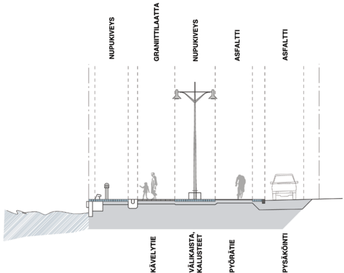
Havainnepoikkileikkaus matkustajasataman pinnoitteiden ja katuvihreän alueista.
