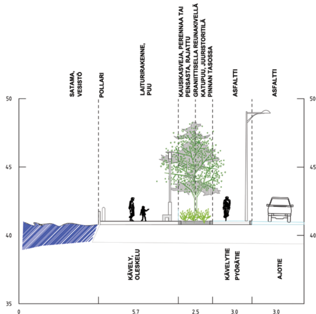
Havainnepoikkileikkaus matkustajasataman pinnoitteiden ja katuvihreän alueista.
