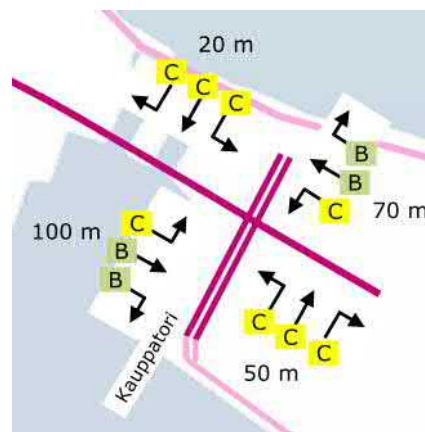
Toimivuustarkastelu 2013. Palveluluokitus ja enimmäisajonopitus liittymäsuunnittain normaalitilanteessa.
