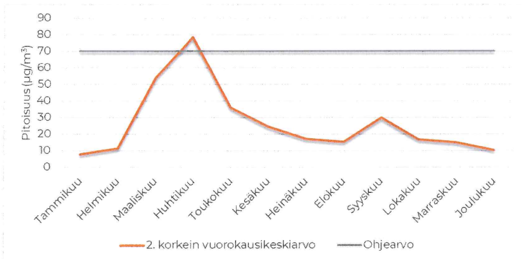
Kuva 13. Hengitettävien hiukkasten pitoisuudet suhteessa kansalliseen vuorokausiohjeeseen Olavinkadulla vuonna 2024.
