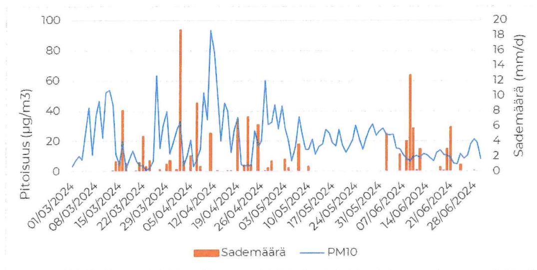
Kuva 29. Hengitettävien hiukkasten ja sademäärän vuorokausikeskiarvot maaliskesäkuussa 2024 Olavinkadulla.
