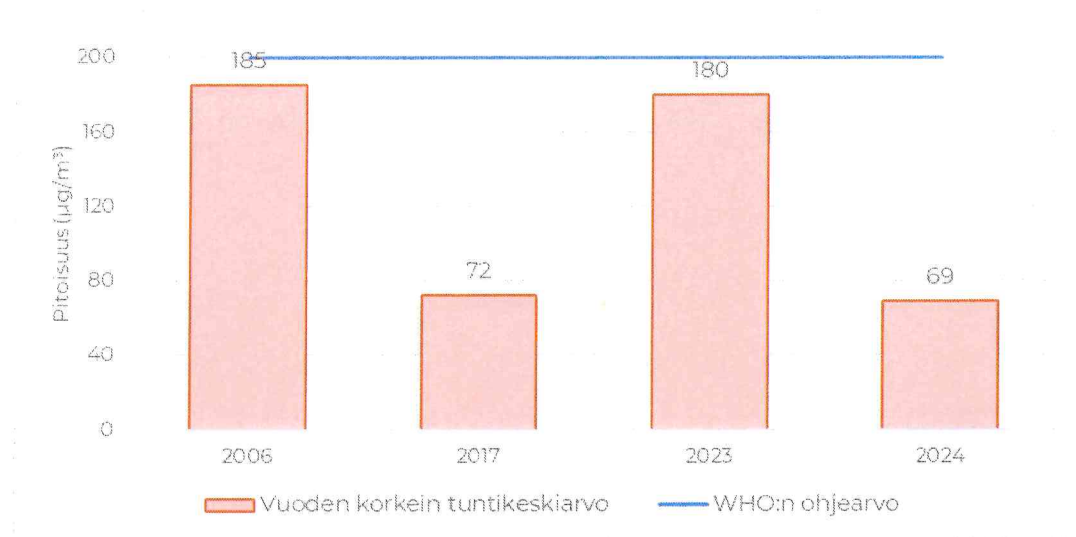
Kuva 24. Typpidioksidin tuntiarvot suhteessa WHO:n ohjearvoon Savonlinnassa vuosina 2006–2024.
