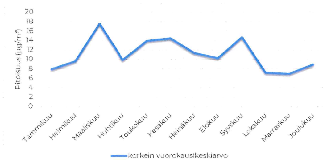
Kuva 19. Pienhiukkasten korkeimmat vuorokausikeskiarvot Olavinkadulla vuonna 2024.
